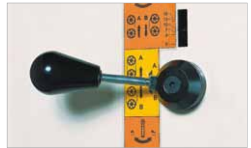
Bandschnellspannhebel und Sägebandeinstellung an der Rückseite der Maschine
