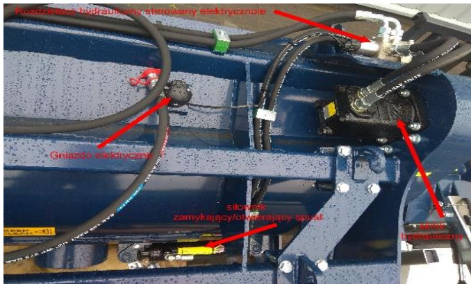
Hydr. System mit Magnetventil
